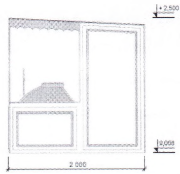
Боковой фасад
