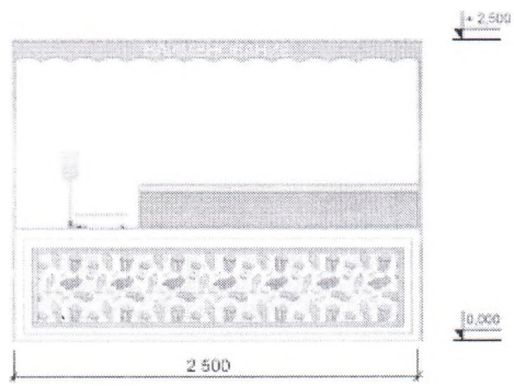
Главный фасад
